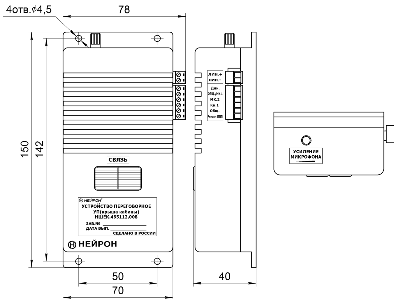
Рис.1 Внешний вид Устройство переговорное «УП(крыша кабины) НШЕК.465112.008
